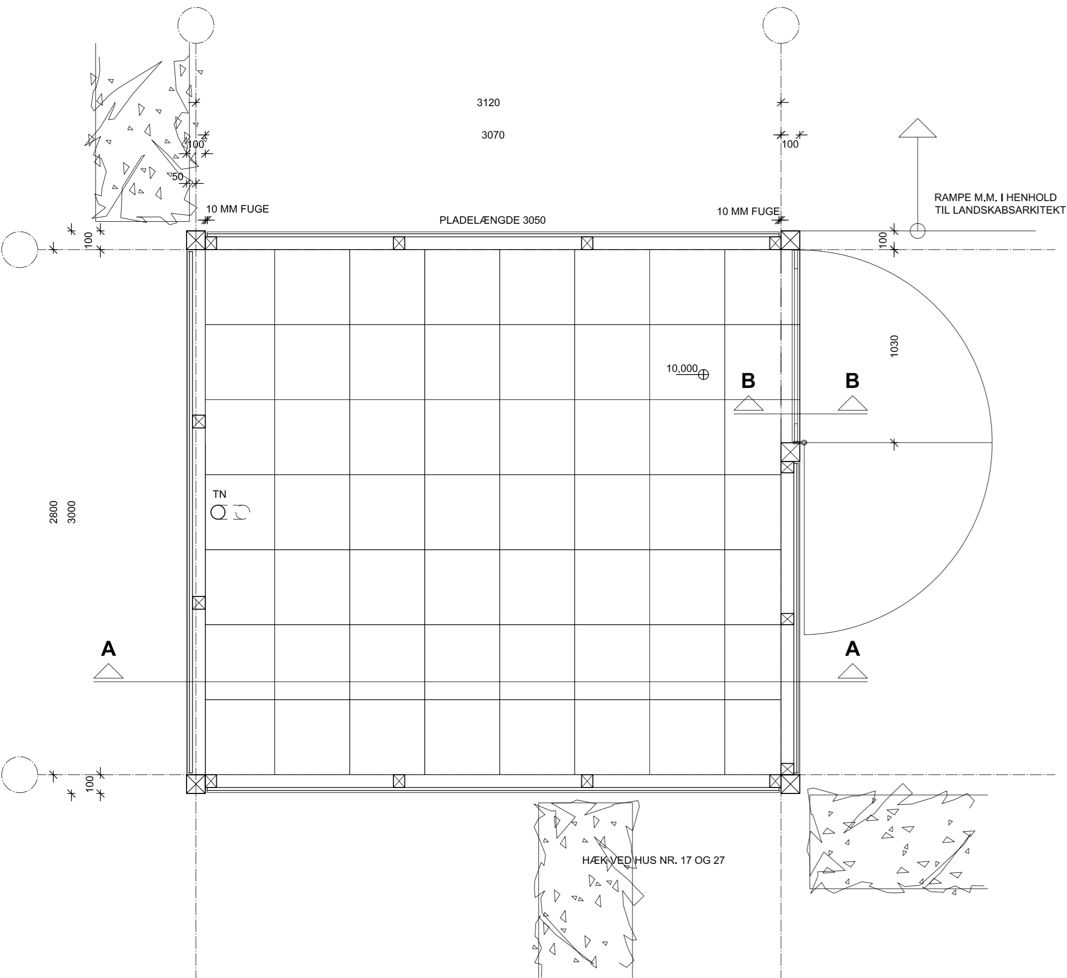
PLAN MÅL 1:20
